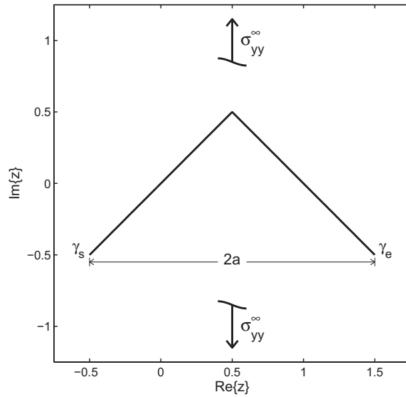
Fig. 9. The V-problem.
